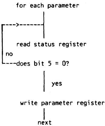
Figure 16. 8271 Parameter Phase Flowchart.
